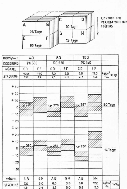
Bild 9. Streuung der Würfeldruckfestigkeit von Probekörpern 20/20/20 cm innerhalb eines Würfels von 40 cm Kantenlänge
