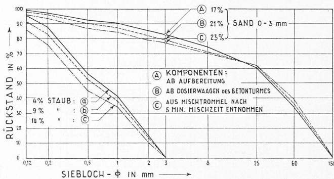
Bild 20. Beispiel für die Staubbildung während dem Transport und dem Mischen der Zuschlagstoffe. Aussiebung von 3 m 3 Material vor und nach einer Mischzeit von 5 Minuten in einem Koering-Kippmischer. Petrographische Qualität: Schieferiger Gneis
