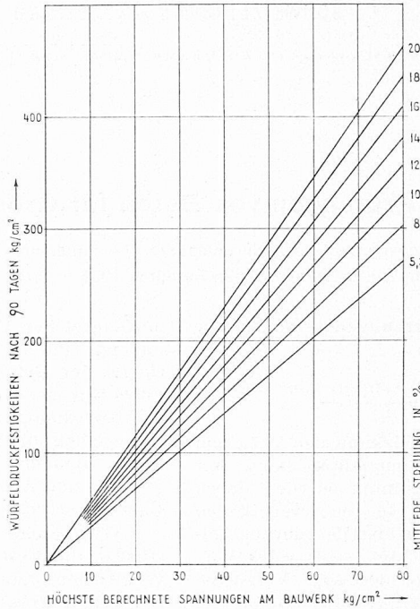
Bild 18. Erforderliche minimale Druckfestigkeit von Betonwürfeln 20/20/20 cm nach 90 Tagen, welche garantiert, dass die Betonfestigkeit bei einer konstatierten Streuung die höchste berechnete Spannung am Bauwerk mit einer Wahrscheinlichkeit von 10^{-7} nie erreicht oder unterschreitet
