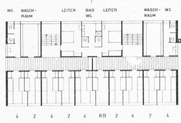
2. OBERGESCHOSS MÄDCHEN
