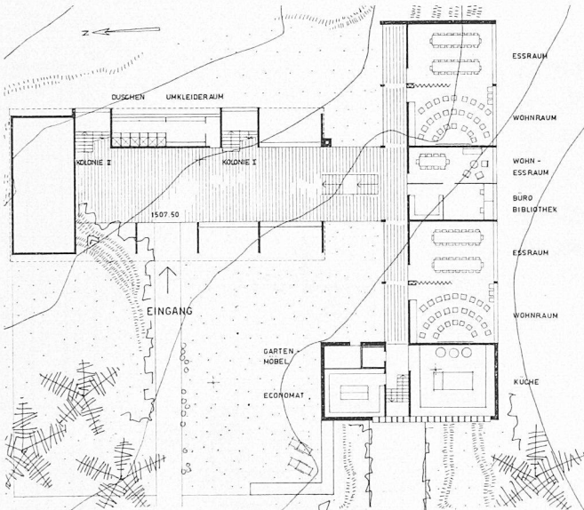
Erdgeschoss 1:600
