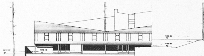
Südansicht
