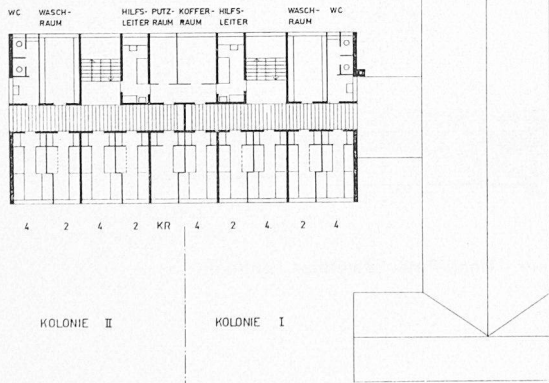
1. OBERGESCHOSS KNABEN
