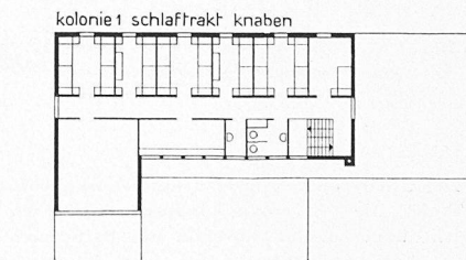
2. Obergeschoss
