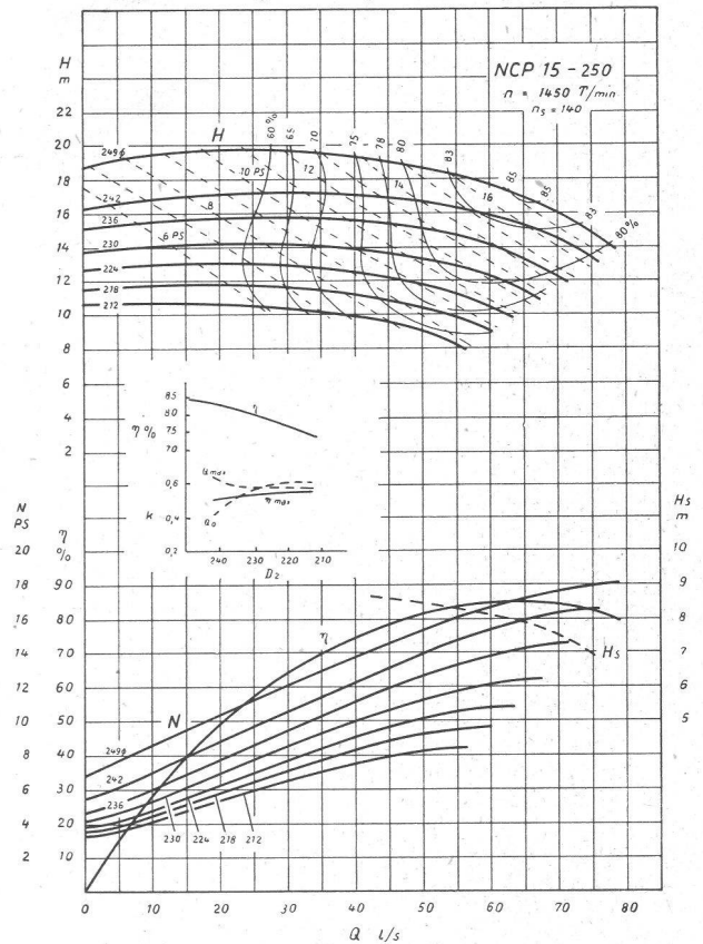
Kennlinien einer Spiralgehäusepumpe mit verschiedenen Laufraddurchmessern
