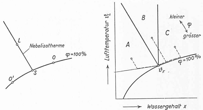
Bild 7. I_x -Diagramm mit Bezeichnung der für die Kaverne Lüftung massgebenden Zustandsfeldern A, B und C
