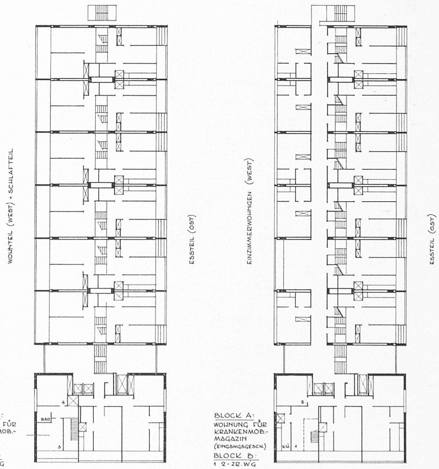
3 1/2 ZIMMERWOHNUNGEN TYP WEST PRO VERTEILSTRASSE: 17 WOHNUNGEN
