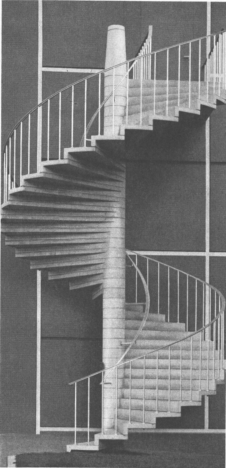
Freistehende Spindeltrappe, Kraftwerk Birsfelden
