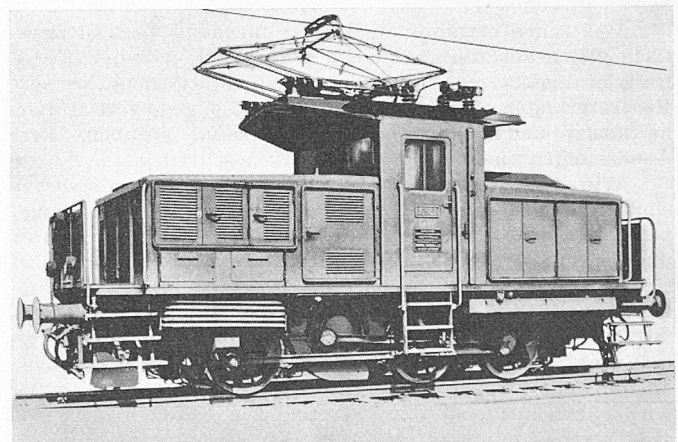
Bild 2. Die Zweifrequenz-Rangierlokomotive Ee3/3II 16502. Die Lokomotiven 16501-06 haben äusserlich praktisch denselben Aufbau.
