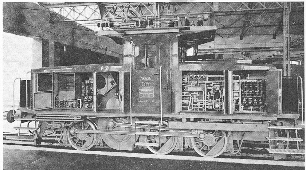
Bild 23 (Mitte). Lokomotiven 16501/02. Elektrische Apparate im hinteren Vorbau
