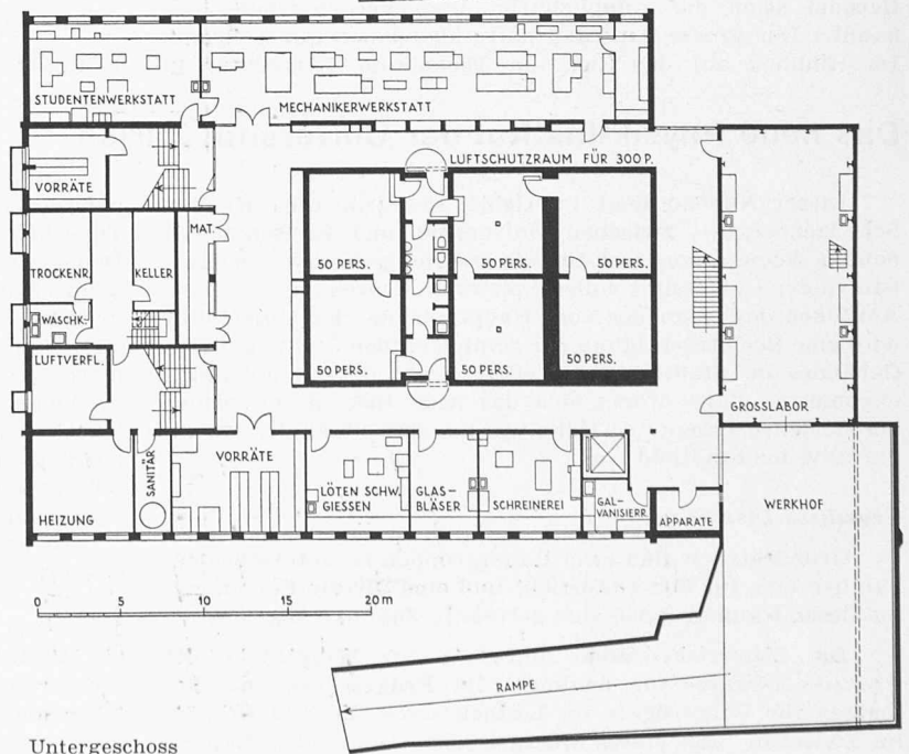
Untergeschoss
