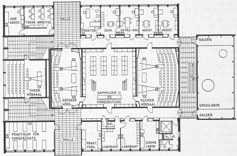
Erster Stock
