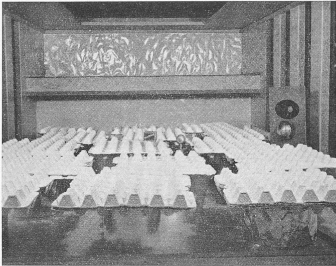
Klanggetreue Nachbildung des Studentenhaussaales in Karlsruhe als Modell im Masstab 1:10 mit Ersatz des Publikums durch präparierte Eierkisteneinsätze. Die Streichholzschachtel bildet ein Grössenmass für den Modellkopp
