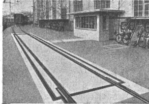
Brückenwaage für Geleisefahrzeuge. Wägefähigkeit 150 000 kg
