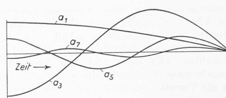
Bild 7. Harmonische Analyse für den Fall mit einem grössten Winkelausschlag von \pm 90^\circ . a_1 ist die mit der Pendelzahl übereinstimmende Kraftkomponente; a_3 die harmonische Kraft dritter Ordnung, die also dreimal so rasch wie die Pendelzahl wechselt, a_5 die harmonische Kraft fünfter Ordnung, a_7 jene siebenter Ordnung
