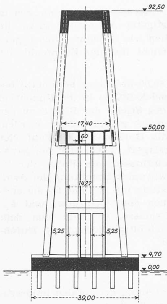
Bild 9. Querschnitt zu Bild 8 in Pfeileraxe, 1:1400
