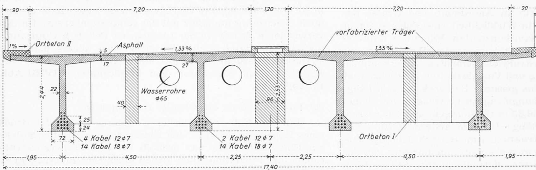
Bild 6. Einhängeträger von 45,95 m in der 85-m-Öffnung, Querschnitt 1:120. Rechtsfallende Schraffur bedeutet, abgesehen vom Plattenbereich, Ansichtsfläche Ortbeton
