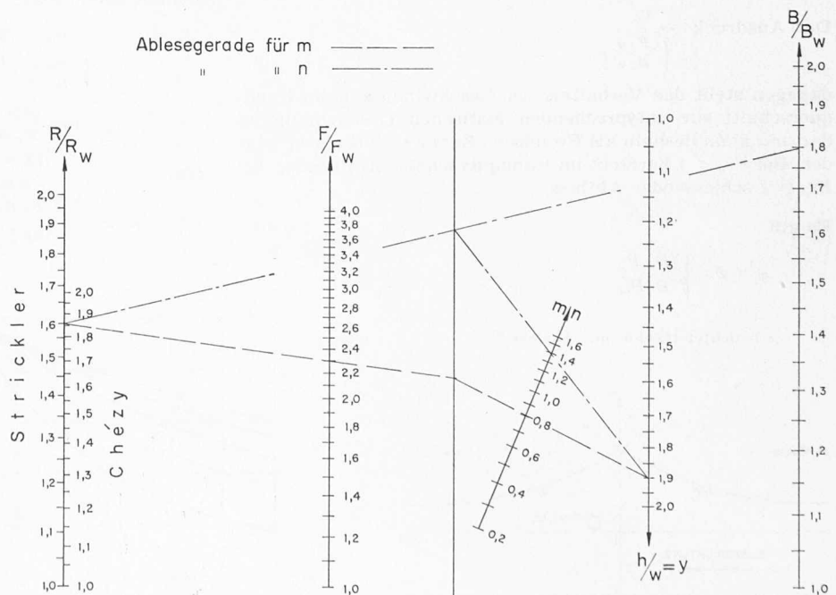
Bild 4. Nomogramm zur Ermittlung der hydraulischen Exponenten.
