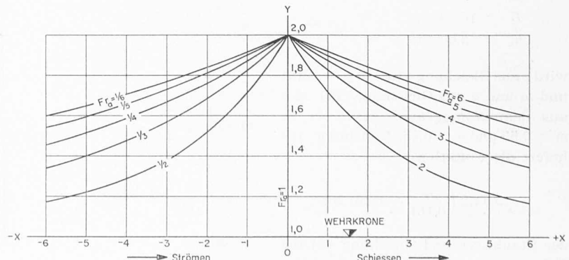
Bild 3. Einfluss der Froudschen Zahl Fr_a auf das Gefälle und die Krümmung der Wasserspiegel (mehrfach überhöhter Längsschnitt)
