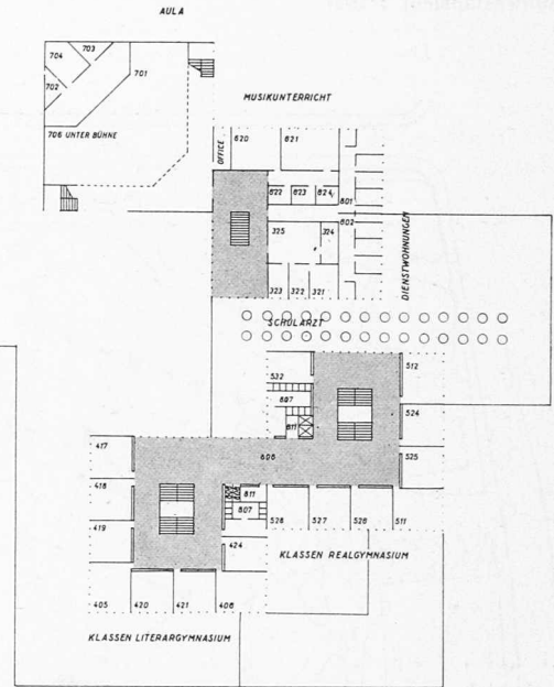
1. Obergeschoss 1:1500
