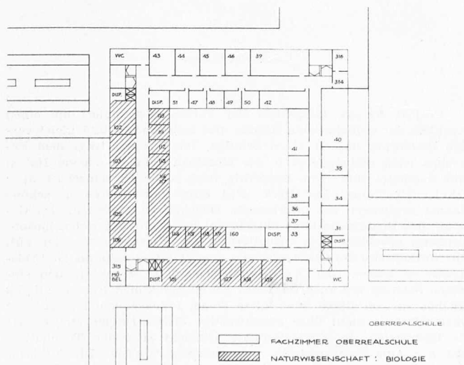
Normalgeschossplan 1:1500
