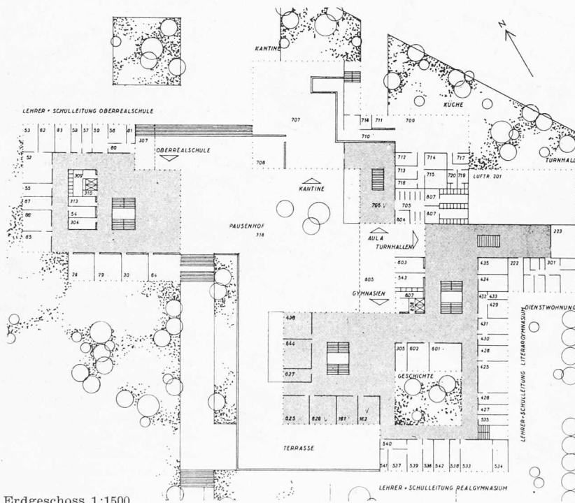
Erdgeschoss 1:1500
