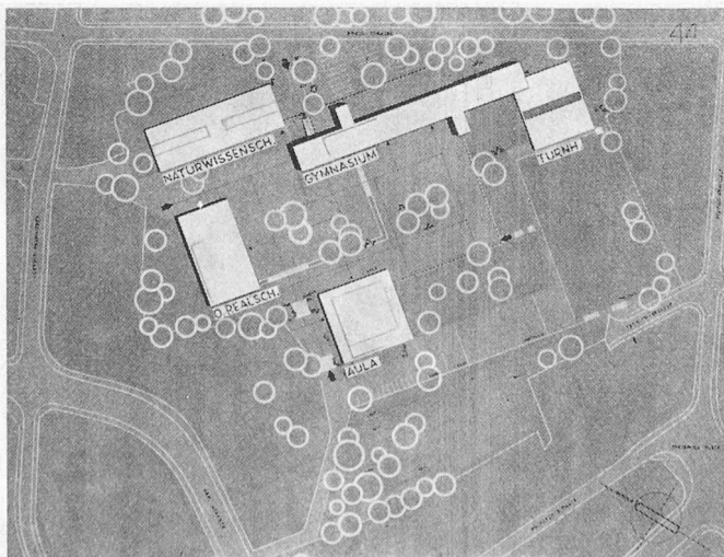
Lageplan 1:4000, 5. Preis
