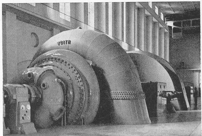
Bild 11. Pumpspeicherwerk Reisch-Rabenleite, Maschinenhalle.
