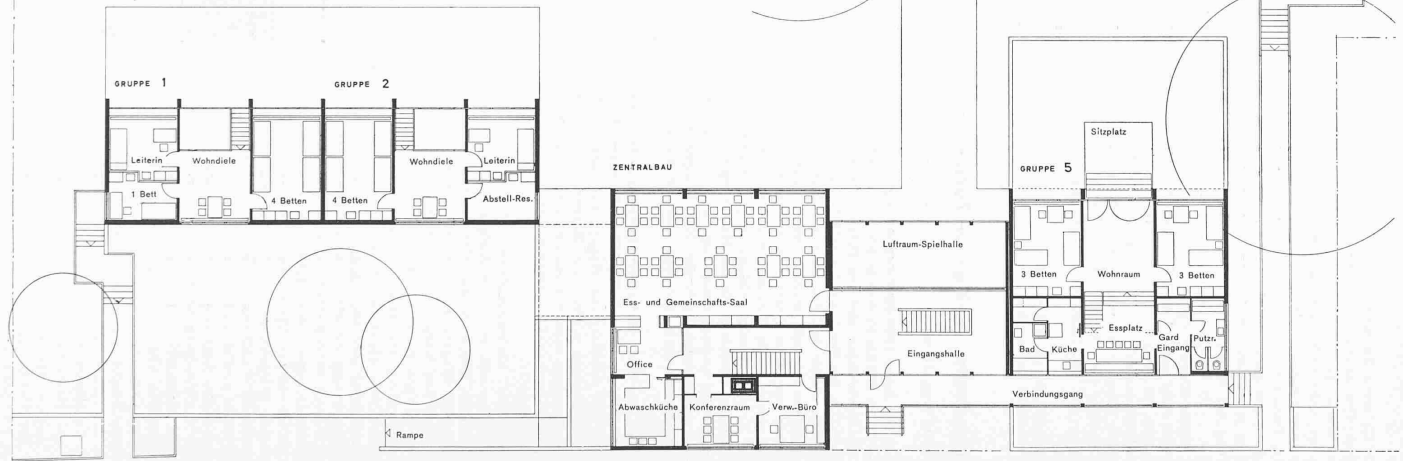
OBERES EINGANGSGESCHOSS
