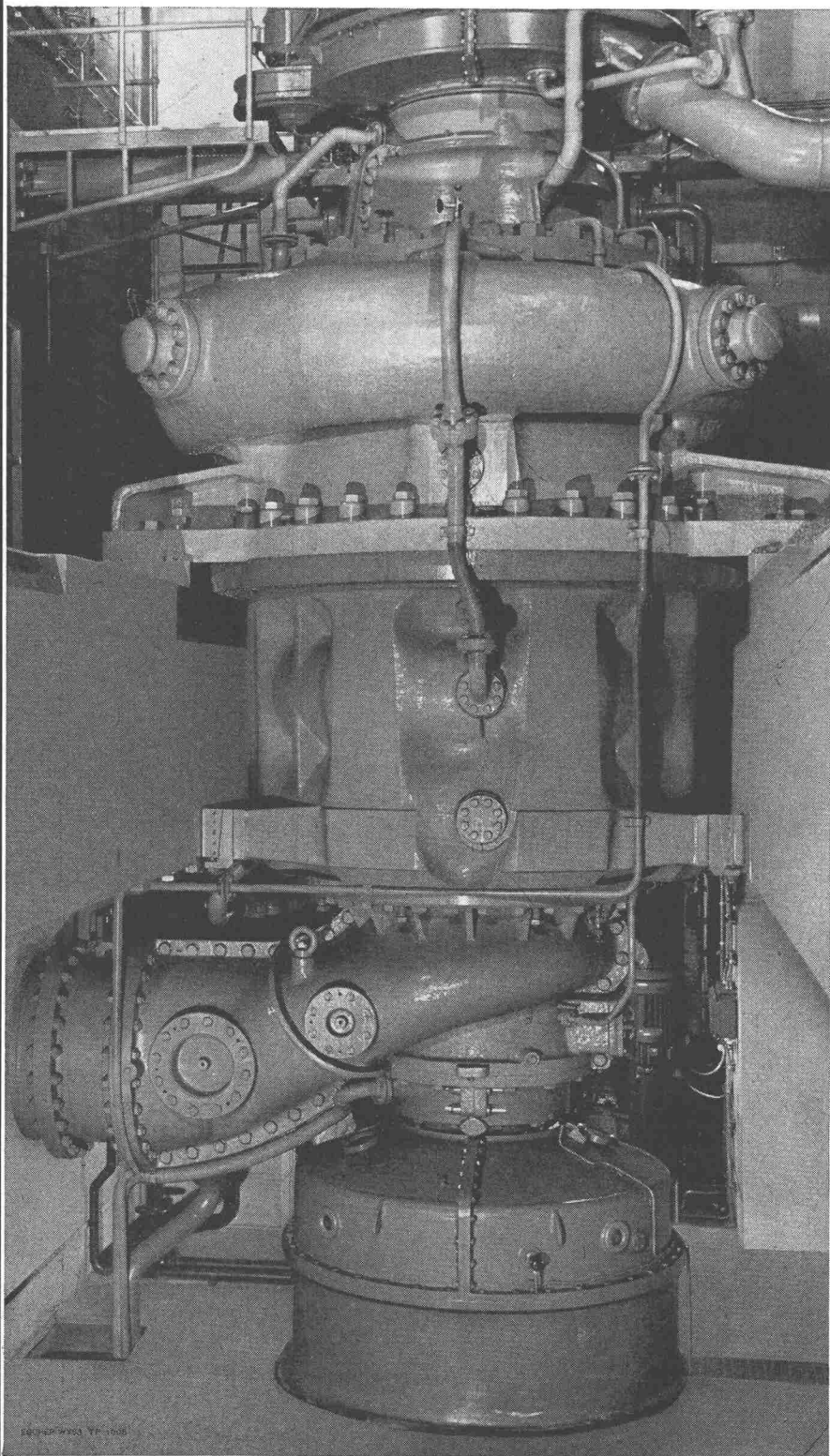
Eine der beiden Speicherpumpen Lünersee; Antriebsleistung 53 820 bis 57 600 PS
