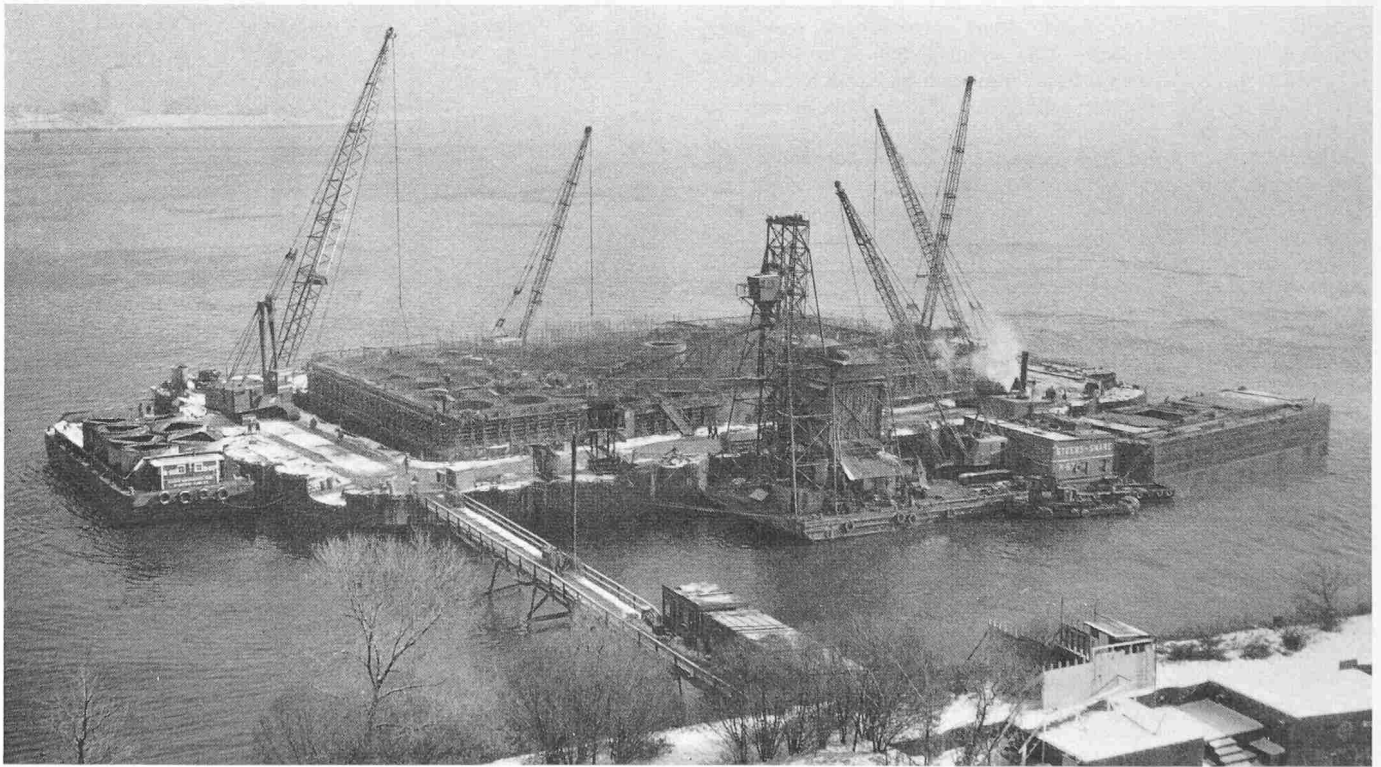
Bild 6. Fundament des Pylons Seite Staten Island, Blick gegen Südosten am 30. Dez. 1960. Plazieren der Schalungen für die elfte Betonieretappe
