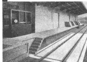
Brückenswaage für Geleise- und Strassenfahrzeuge, Wägefähigkeit 80 000 kg, mit Laufgewichtsbalken und autom. Schnellanzeige
