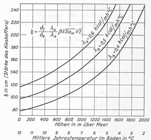
Bild 18. Zunahme der Kieskofferstärke mit abnehmender mittlerer Jahrestemperatur bzw. mit zunehmender Meereshöhe für verschiedene Wärmeleitfähigkeiten des Koffermaterials bei einer Temperatur im Kühlröhrensystem von -8^\circ\text{C} und einer Temperaturleitfähigkeit von 0,0020 \text{ m}^2/\text{h} , einer Wärmeleitfähigkeit des Bodens von 1,2 \text{ kcal/mh}^\circ\text{C} und einer Betriebsdauer von 3600 Stunden
