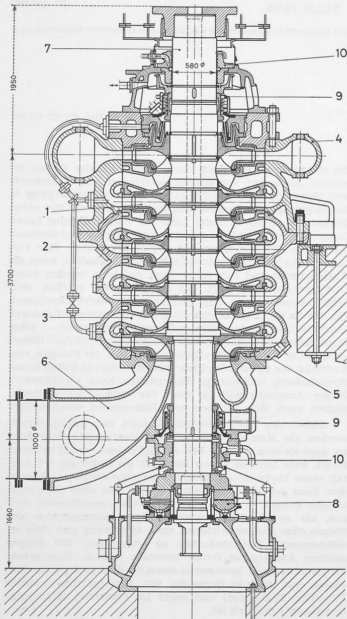
Bild 3. Speicherpumpe Lünernersee in einflutiger, fünfstufiger Ausführung
