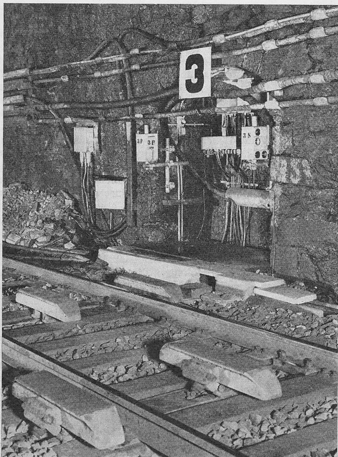
Bild 5. Blockstation 3 im Tunnel. Am Gleis die Streckengeräte für die automatische Zugsicherung (Gleismagnete) für beide Fahrriichtungen. An der Tunnelwand von rechts nach links: Blocksinal 3S Fahrriichtung nach Göschenen, Kabelverteiler, Blocksinal 3P Fahrriichtung Airolo, Telefonsignal, Schwachstromkabelkasten
