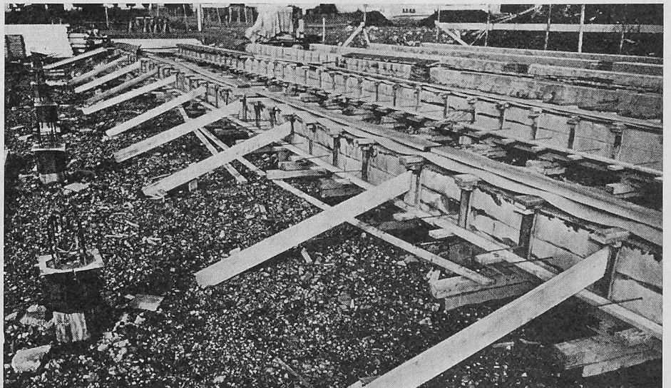
Bild 8, Betonieren der Pistenräger
