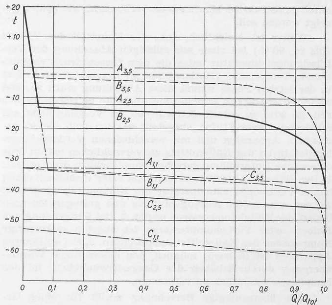
Bild 3. Temperaturverlauf bei der Chlorverflüssigung in einem vertikalen Rohrbündel in Abhängigkeit der verhältnismässigen Wärmeumsätze. A dem Gesamtdruck entsprechende Verflüssigungstemperatur. B Tatsächliche Verflüssigungstemperatur des Chlorgases. C Temperatur des verdampfenden R 12. Die Indices geben die Gesamtdrucke an
