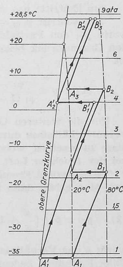
Bild 1. Zwei- und dreistufige Verdichtung von Chlorgas im i, \lg p -Diagramm
