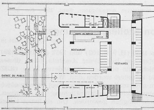
2 e NIVEAU : ENTREE DU PARC - RESTAURANT - VESTIAIRES
