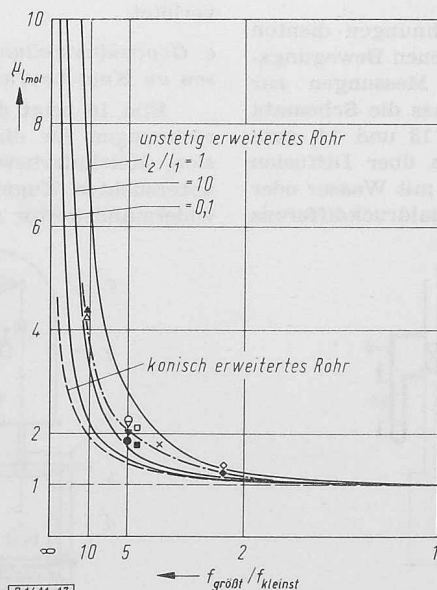
Bild 18. Knudsen-Molekularbewegung
