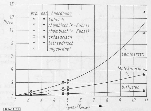
Bild 16. Widerstands factor \mu_{l,Erw} für Porenverengung bzw. Porenverengung von Kugelhauferwerken in Abhängigkeit vom Flächenerweiterungsverhältnis f_{\text{groest}}/f_{\text{kleinst}} für verschiedene Bewegungsarten
