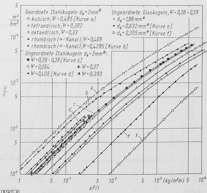
Bild 6. Luftdurchlässigkeit in Abhängigkeit vom Druckgefälle. d_k : Kugeldurchmesser, \psi Porosität des Haufwerkes
