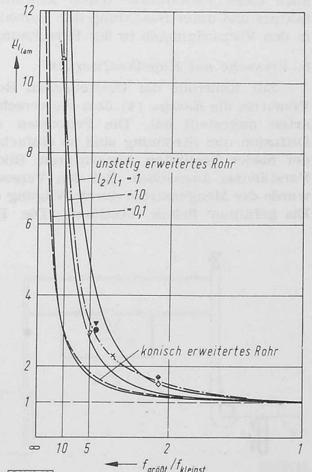
Bild 19. Laminarströmung
