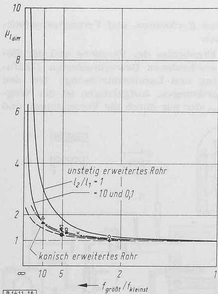
Bild 17. Stefansche Diffusion
