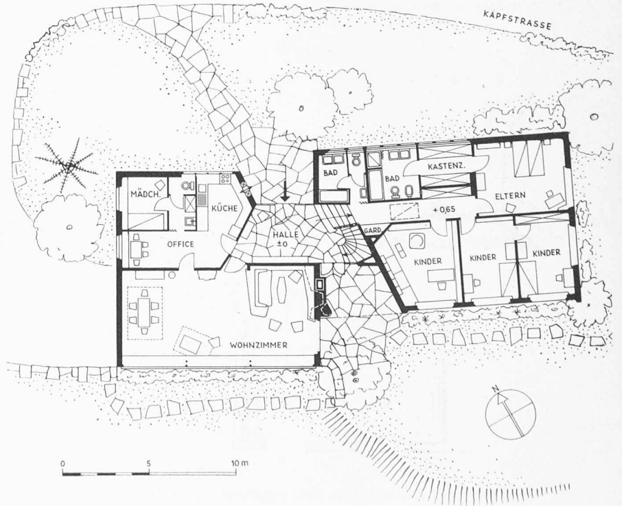
Erdgeschoss Masstab 1:300
