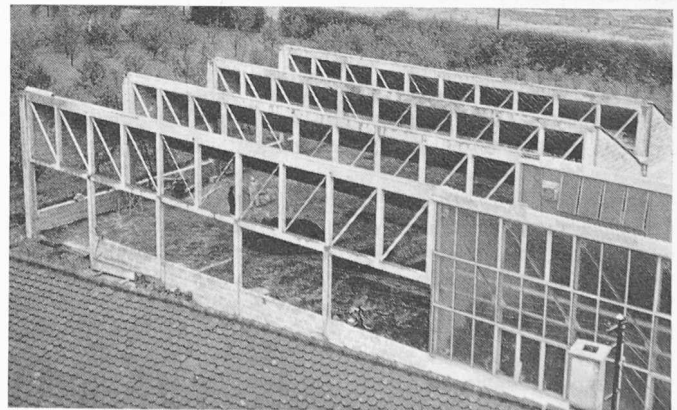
Bild 15. Shedhalle mit Fachwerkbindern in der Fensterfläche
