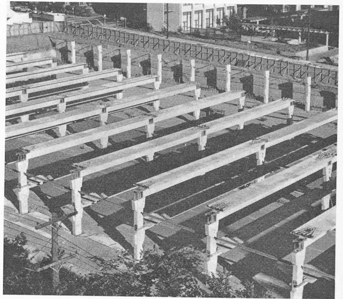
Bild 28. Zweigeschossige Universitätsgarage in Berkeley, Cal., mit Lin-T-Elementen
