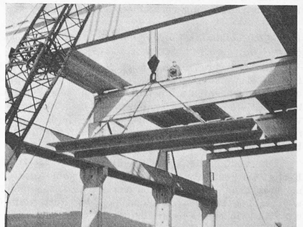
Bild 7. Versetzen der grossformatigen Dachelemente
