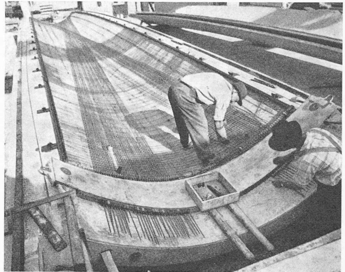
Bild 23. Fertigung der HP-Schalen im Spannbett
