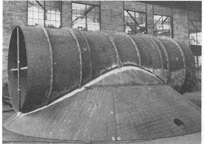
Druck- und Verteilung «Linthal». Drosselrohr mit Uebergangskonus zu Wasserschloßpanzerung. Innen- \phi 3000 mm, Konus- \phi 8250 mm, Wandstärke 10 mm
