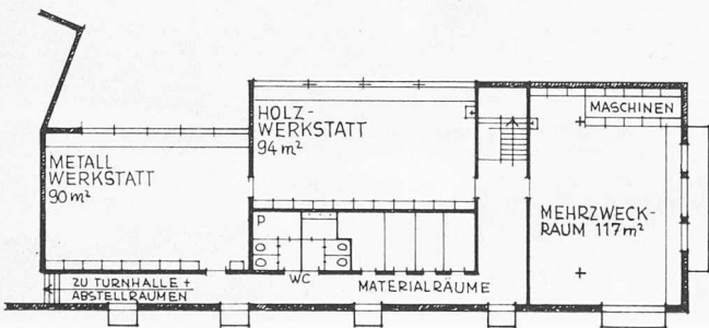
Untergeschoss 1:400
