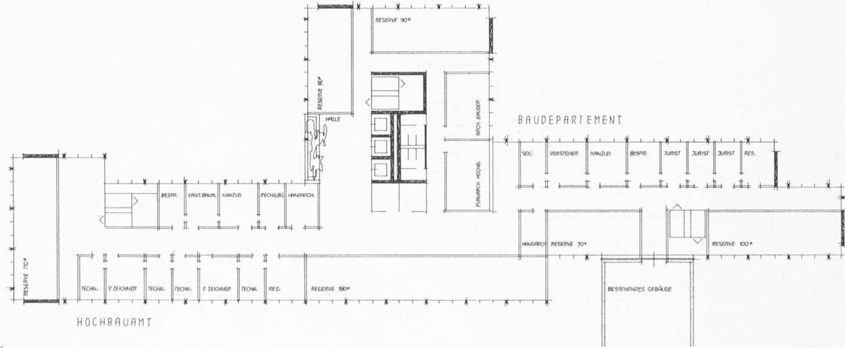
2. GESCH. Grundrisse 1:700
