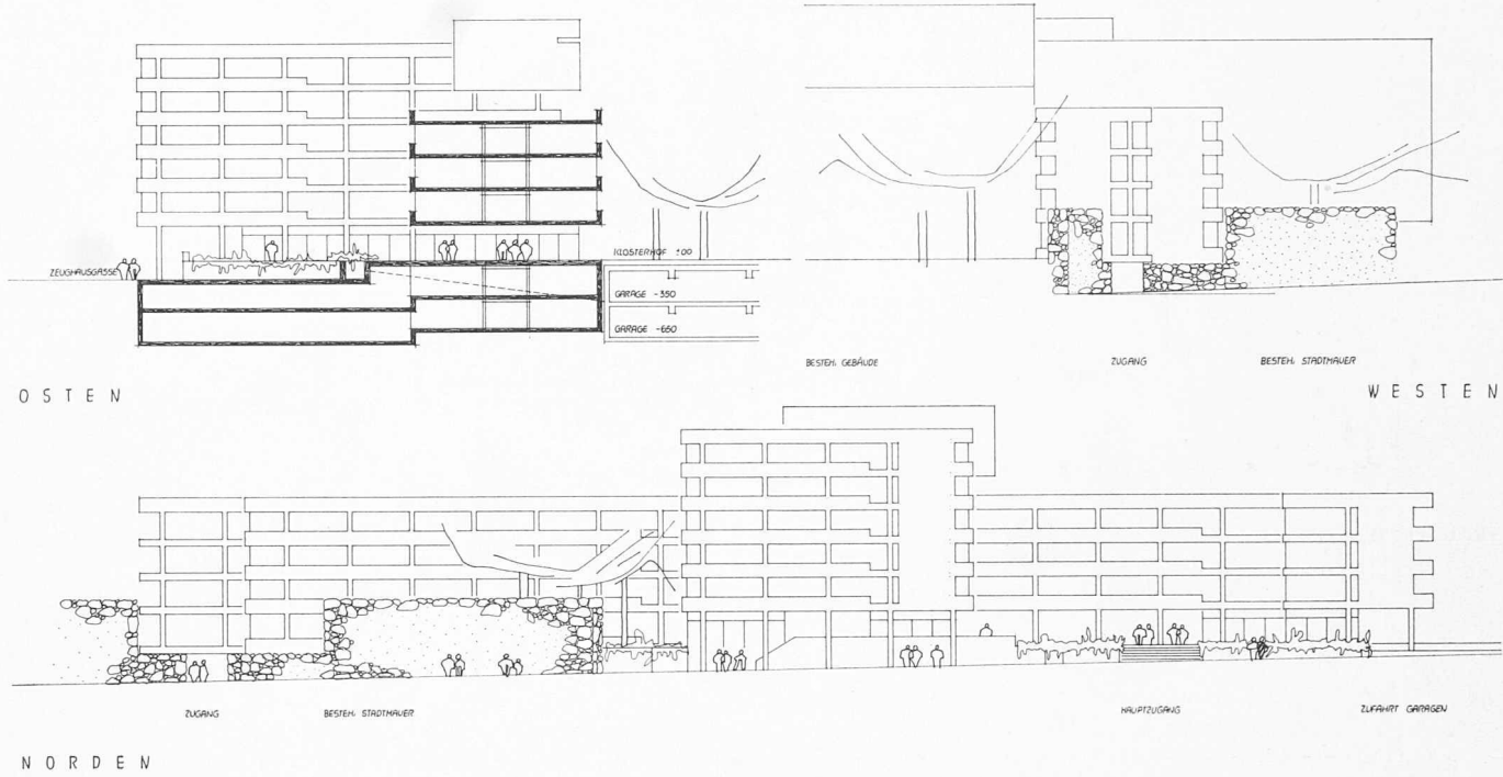
Fassaden 1:700
