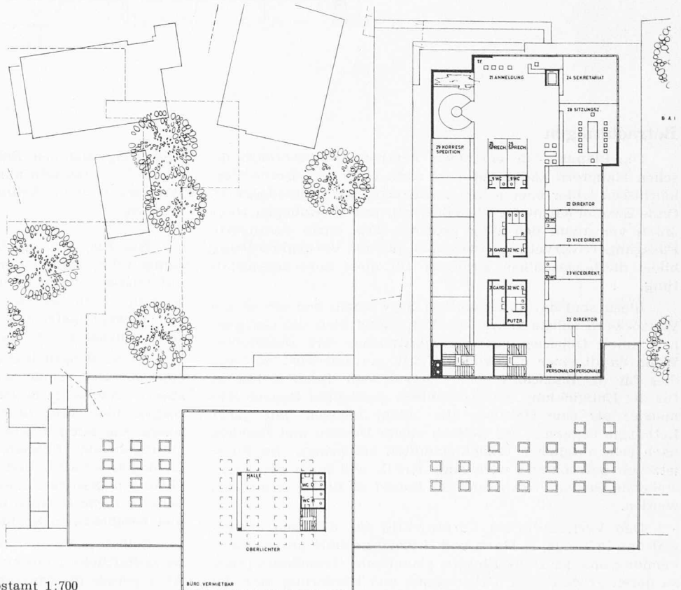
Rechts: 2. Obergeschoss Bank 1:700
