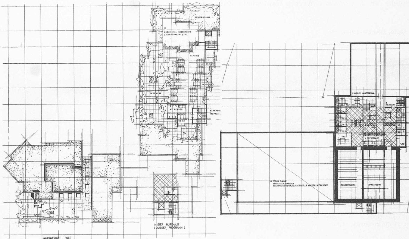
3. Obergeschoss 1:700
