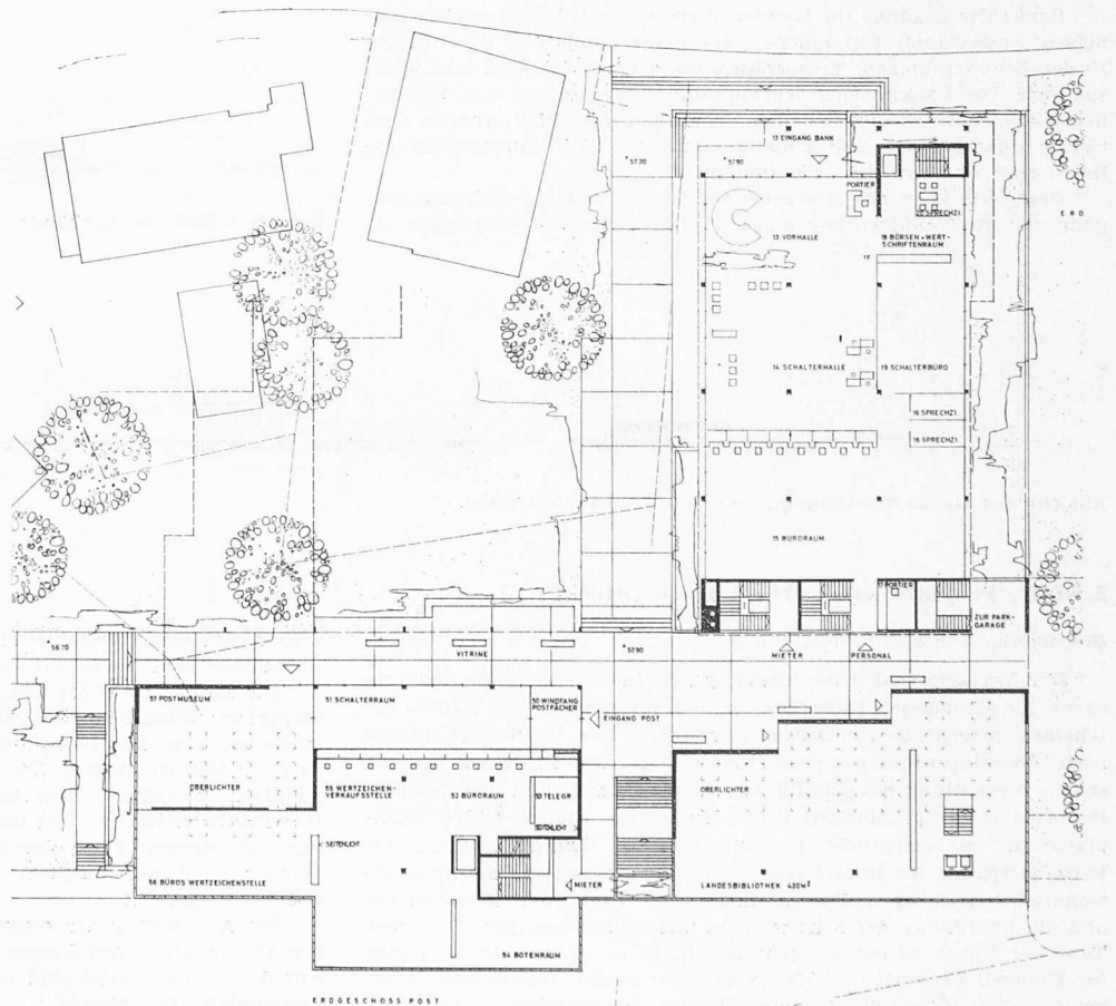
Erdgeschoss 1:700, Bank und Postamt
