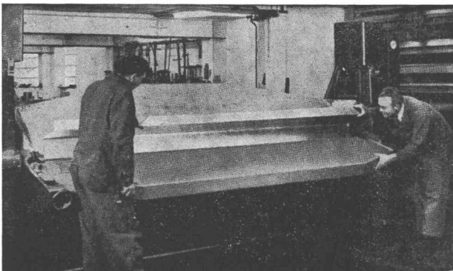
Vorderansicht der vollhydraulischen Abkantmaschine. Ihr wesentlichster Vorteil besteht in der vorwählbaren vollautomatischen Programmsteuerung acht verschiedener Blechabwinkelungen.
