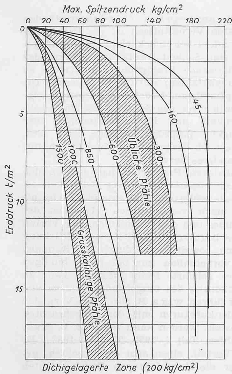
Bild 14. Abhängigkeit des spez. Spitzwiderstandes eines Pfahles von Ueberlagerungsdruck und Durchmesser
