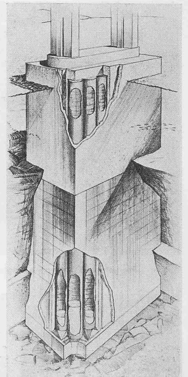
Bild 8. Tajobrücke, Pfeiler abgesenkt
