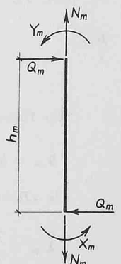
Bild 6. Schnittkräfte des Stiels
