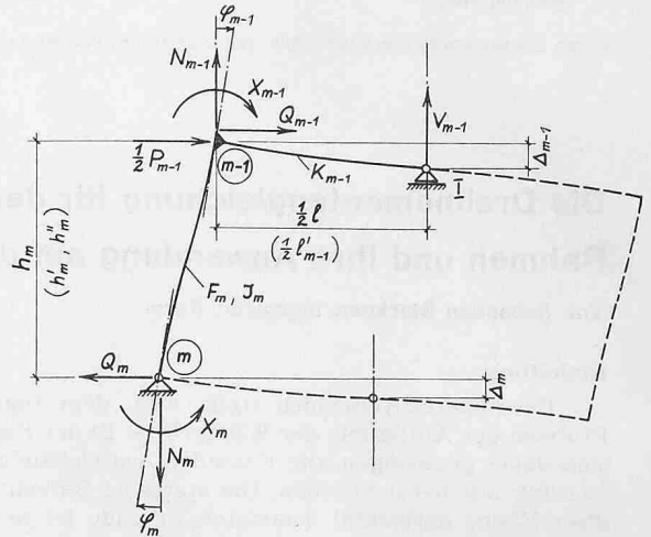
Bild 3. Einhütiger Rahmen
