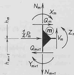
Bild 2. Schnittkräfte am Rahmenknoten
