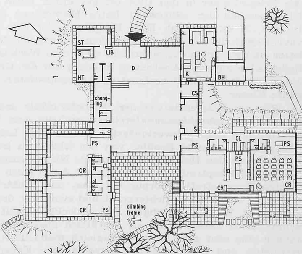
Grundriss der oben genannten Schule. Typisch sind die zentrale Mehrzweckhalle und die gegliederten, mit eigenen Eingängen versehenen Klassenräume. BH = Boiler, CR = Klasse, CL = Garderobe, CS = Hauswartbüro, D = Speisesaal, H = Mehrzweckhalle, HT = Hausvorstand, K = Küche, LIB = Bibliothek, PS = Werknische, S = Material, ST = Lehrer.
