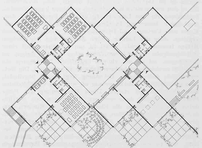
Schulhaus «Riedenhald», Zürich, Primarstufe. Architekten R. Gross, H. Escher und R. Weilenmann. Zusammenfassung von je zwei Klassen zu einer Gruppe mit eigenem Vorplatz, der von manchen Lehrern zur Isolierung einzelner Schüler in den Unterricht einbezogen wird. Die Freilichtunterrichtsplätze können ohne Beeinträchtigung benachbarter Klassen benützt werden.
