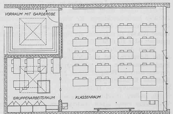
Schulhausprojekt Allenwinden, Baar; Arch. W. Christen, Grundriss der aus Klassenzimmer, abtrennbarem Gruppenraum und Garderobenvorraum bestehenden Klasseinheit
