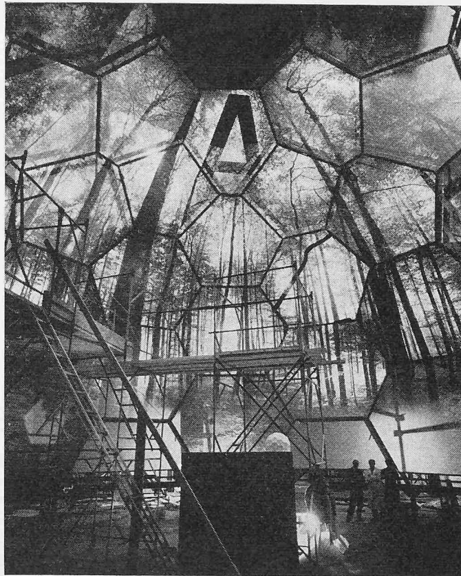
Stahlgerüst und Laufsteg zur Befestigung der Projektoren mit ihren Spiegeln
