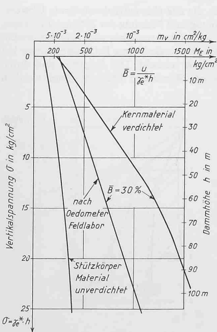
Bild 17 (links). Kompressibilität des Stützkörper- und des Kernmaterials, gemessen am Göschenalpdamme.
