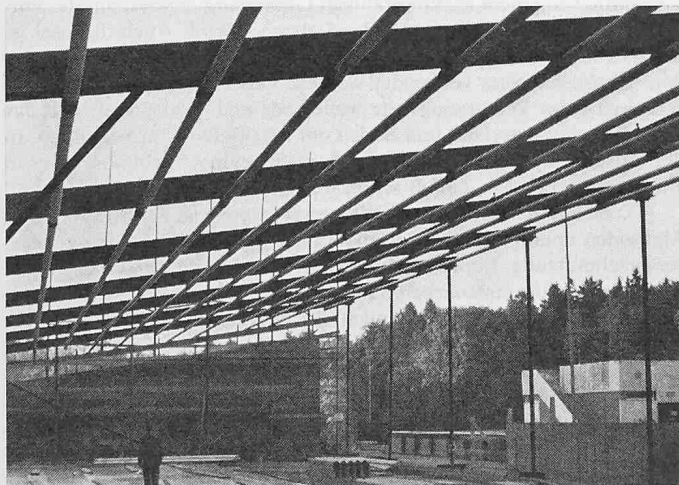
Bild 13. Aufrichten der Stahlkonstruktion
