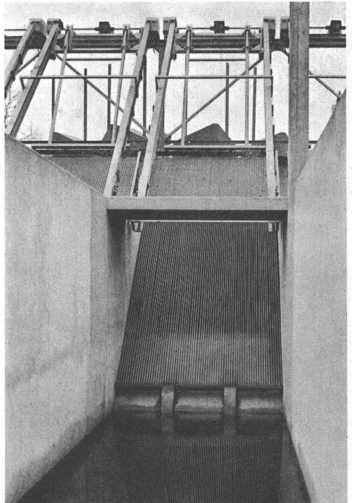
Einlaufrechen mit automatischer Reinigung
