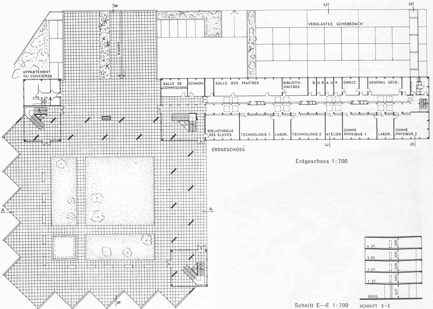
SCHNITT E-E
