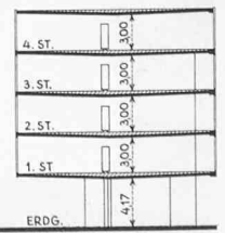
SCHNITT E-E
