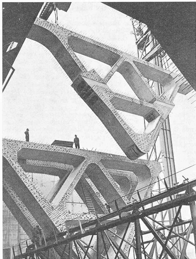
Bild 29. Osterscheldebrücke, Holland. Hohlkastenstücke wurden an stählerne Fachwerkbrücke angehängt und zusammengespannt
