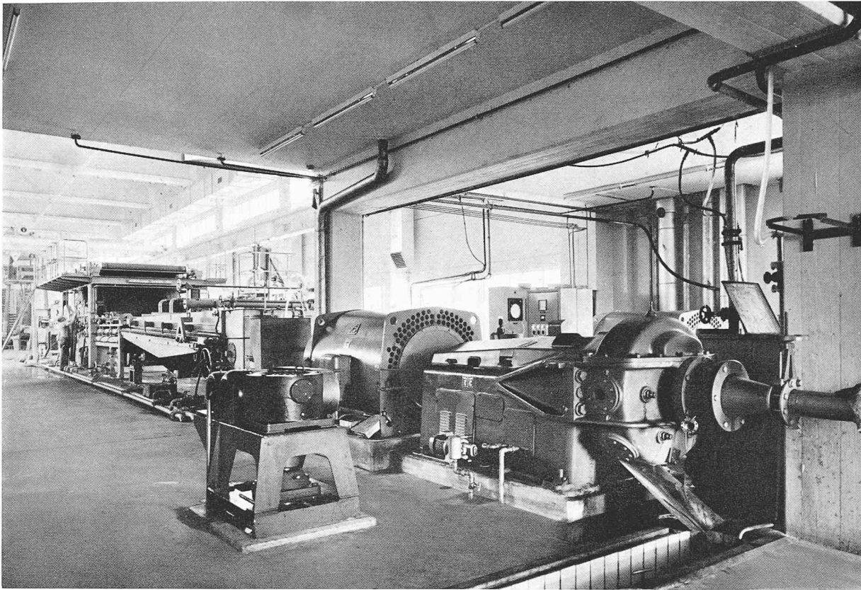
Bild 6. Stoffaufbereitung (6, 7, 9)
