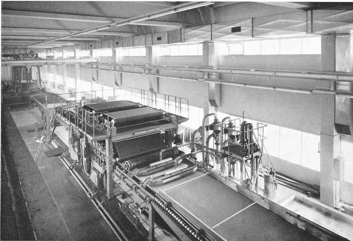
Bild 7. Entwässerungsmaschine (9)
