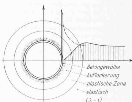
Bild 8. Stabilisierung durch Gewölbe. Bei sprödem Gebirge sind die Verformungen mit Rissen und entsprechender Auflockerung am Ausbruchinnenrand begleitet. Durch die Belastung des Betongewölberings wird die Spannungsspitze abgebaut und ausgerundet. So kann die plastische Zone im Gebirge stabilisiert werden.
