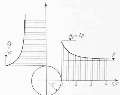
Bild 3. Bei gleicher Horizontal- wie Vertikalspannung verteilen sich die Spannungen um den ganzen Tunnelumfang gleichmässig mit einer Spannungsspitze am Innenrand von 2 p . \lambda = 1 , q = p , m = 2 , \nu = 0,5
