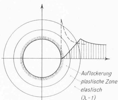
Bild 7. Geschieht die Spannungsumlagerung im Gebirge nicht plastisch, sondern durch Bruchverformungen, so kann der Fels am Ausbruchrand keine Spannungen übernehmen. Es entsteht eine Auflockerungszone und die Spannungen verlagern sich noch weiter ins Bergesinnere.
