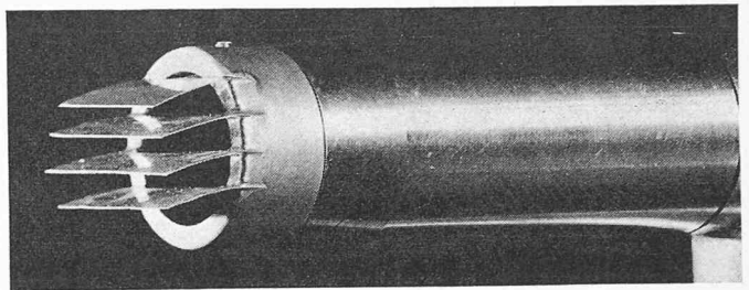
Bild 15. Treibstrahldüse mit Strahlablenkung durch Gitter
