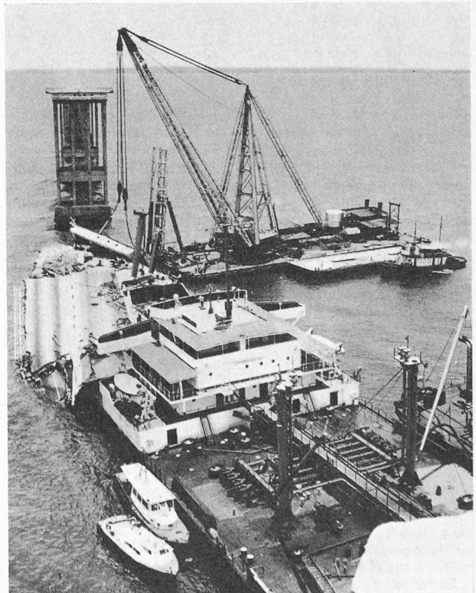
Bild 6. Beseitigen der Trümmer vom Deck des Tankers
