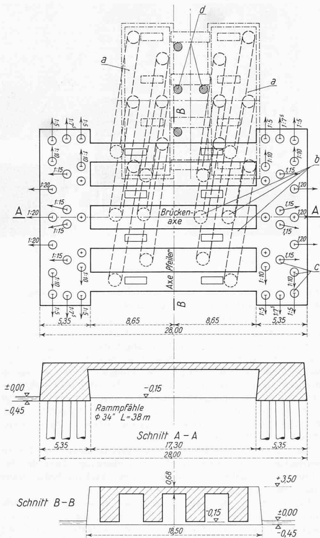
Bild 10. Neue Gründung Pfeiler 31, Masstab 1:450. a = alte, verschobene Pfahlkopfplatte, b = alte, umgebrochene Bohrpfähle, c = Rammfähle \phi 34", L = 38 m, d = Sicherungspfähle für die abgestürzte und verschobene Pfahlkopfplatte
