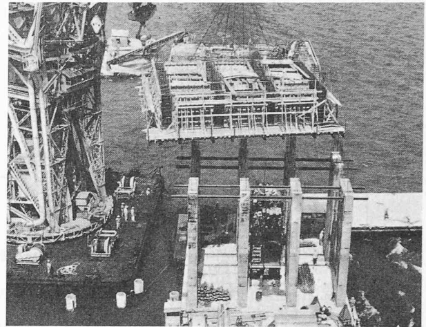
Bild 13. Pfeiler 31, Einsetzen des Querträgeregitters mit Schalung und Bewehrung
