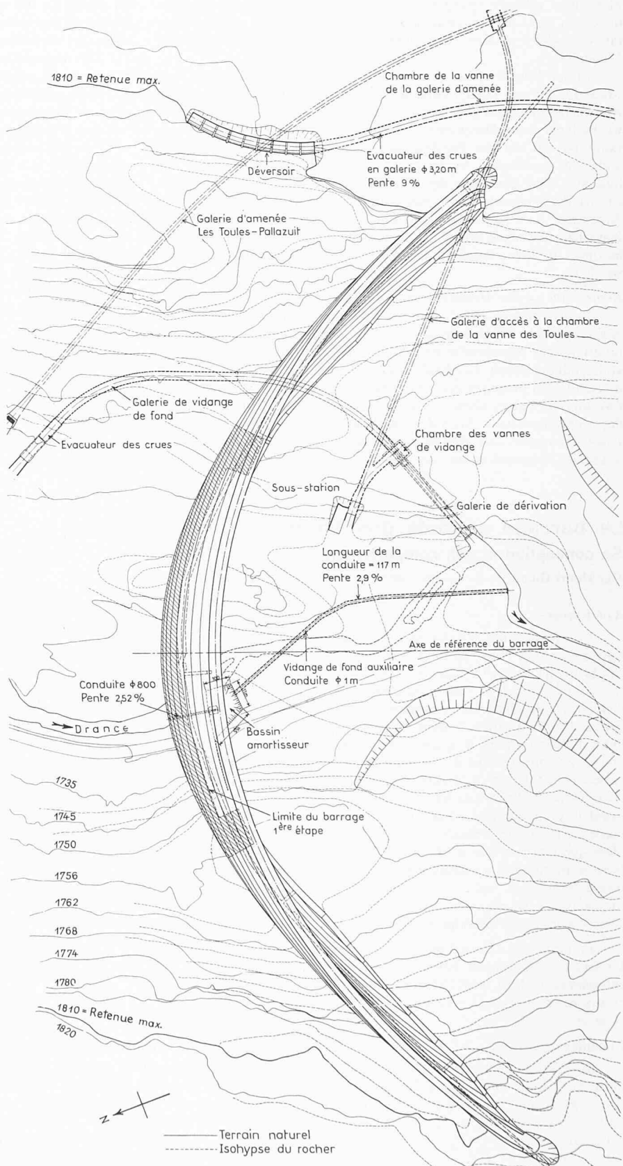
Fig. 1. Vue en plan du barrage des Toules. Echelle 1:2000
