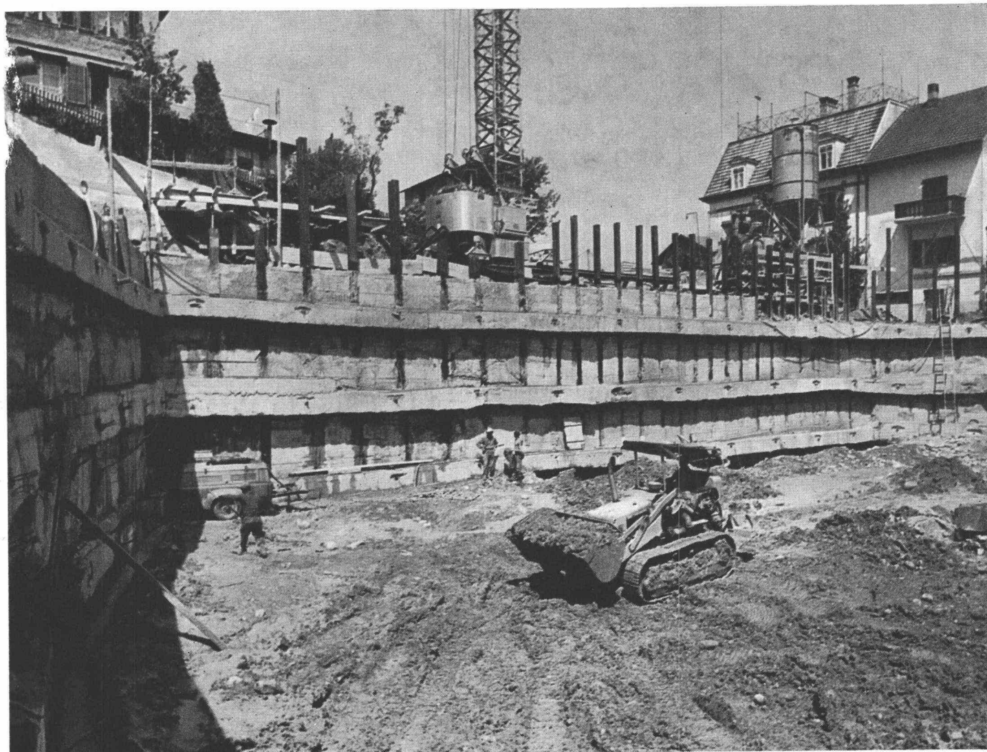
Sprissungsfreie Baugrube
