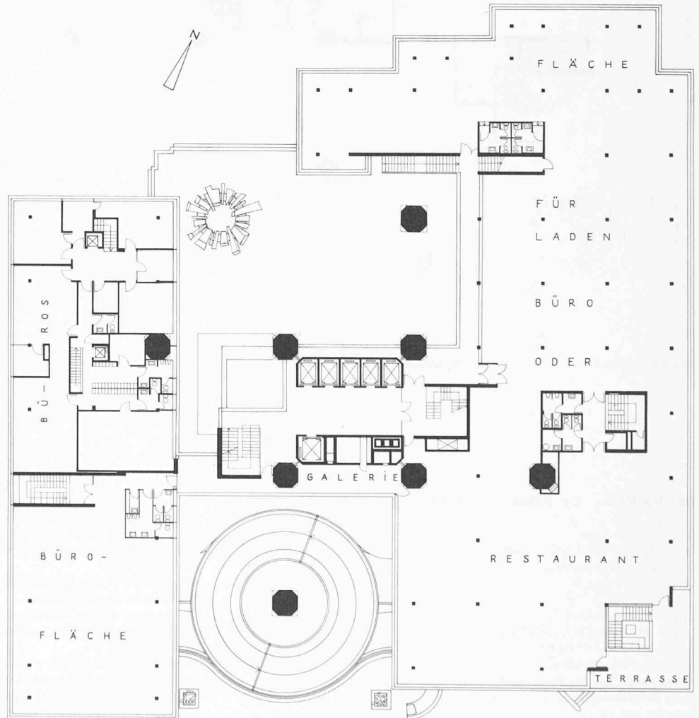
Bild 11. Erstes Obergeschoss 1:500 mit Draufsicht Eingangshof
